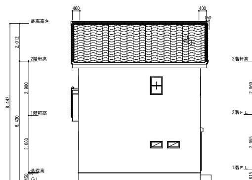
東側 立面図 S:1/100
