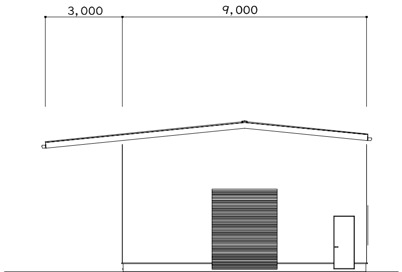
南 立面図
