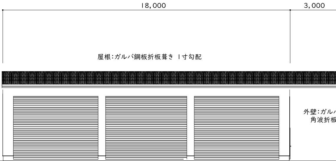
西 立面図
