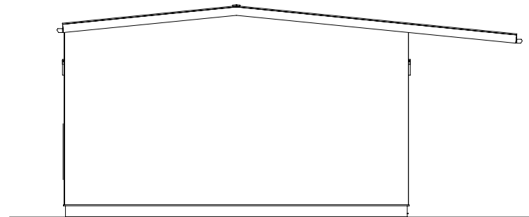
北 立面図
