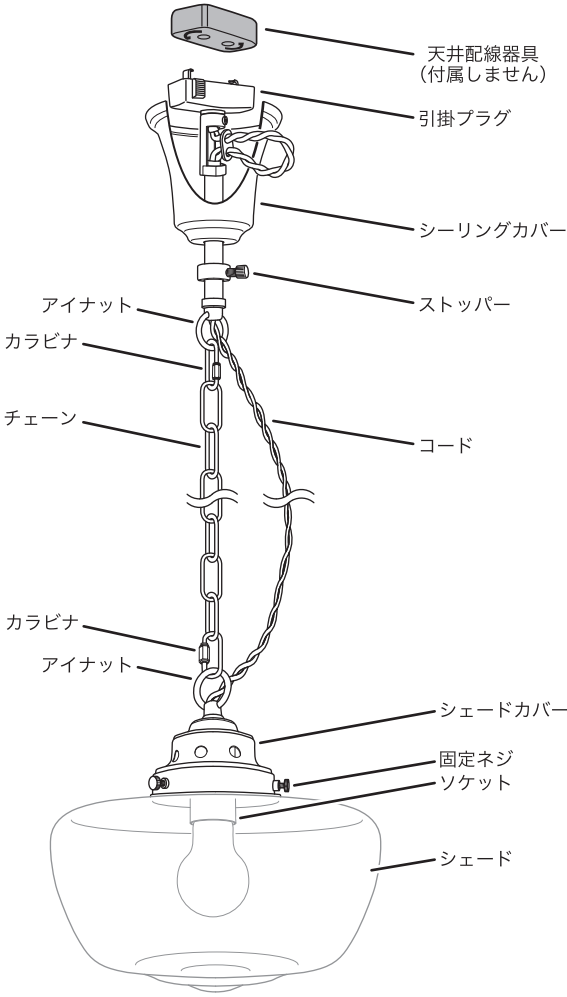
※イラストは MLA-541 のシェードになります
