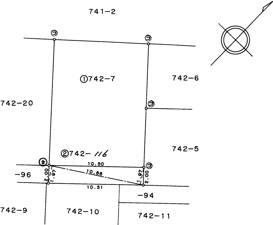
三斜求積表
