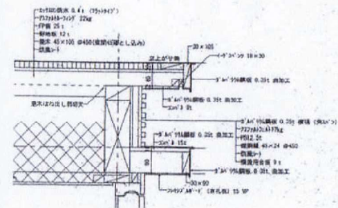
野光部 (C部) 詳細図 1:10
