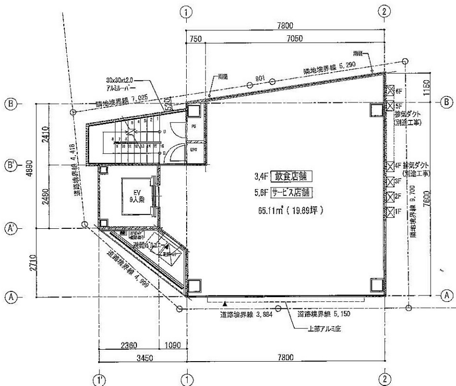
3~6階平面図
