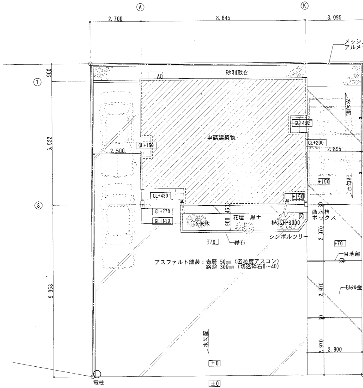
【外構図 1/100】
