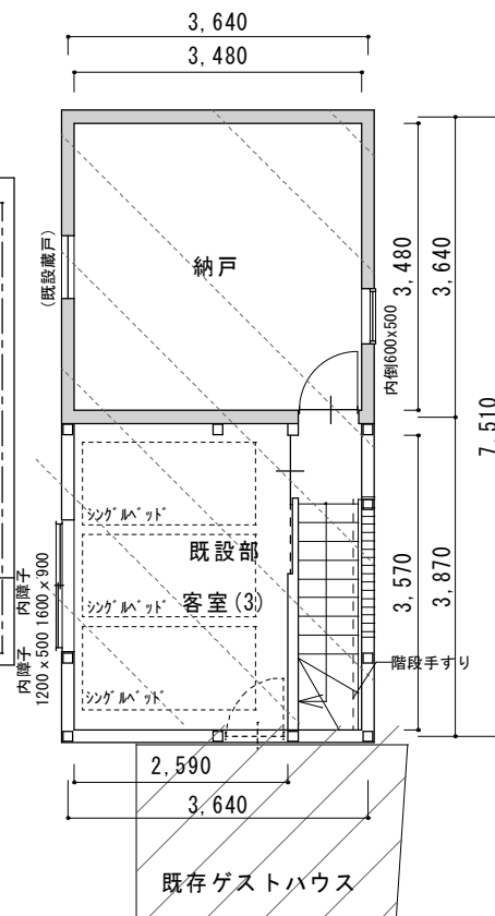
2階平面図 1/100
