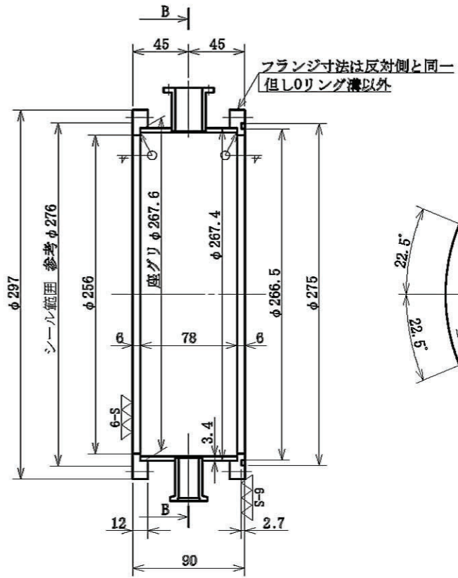
A-A断面
