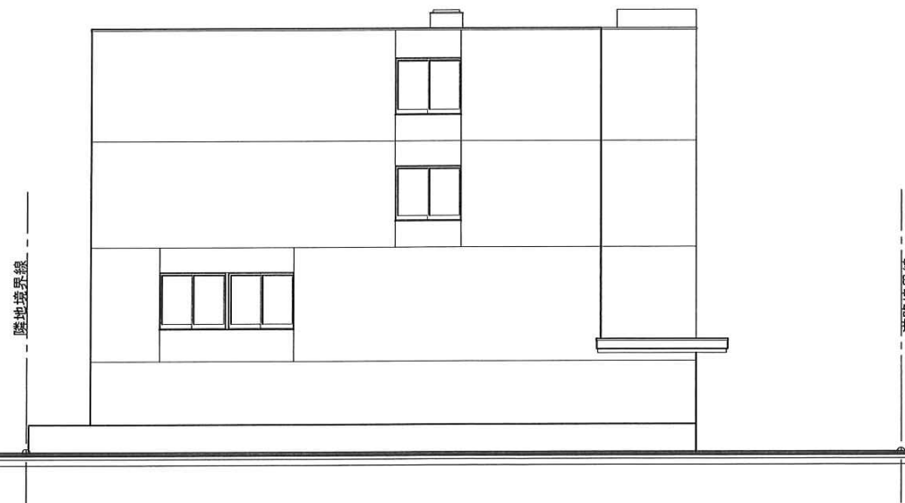
北立面図
