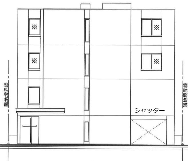
西立面図(正面)
