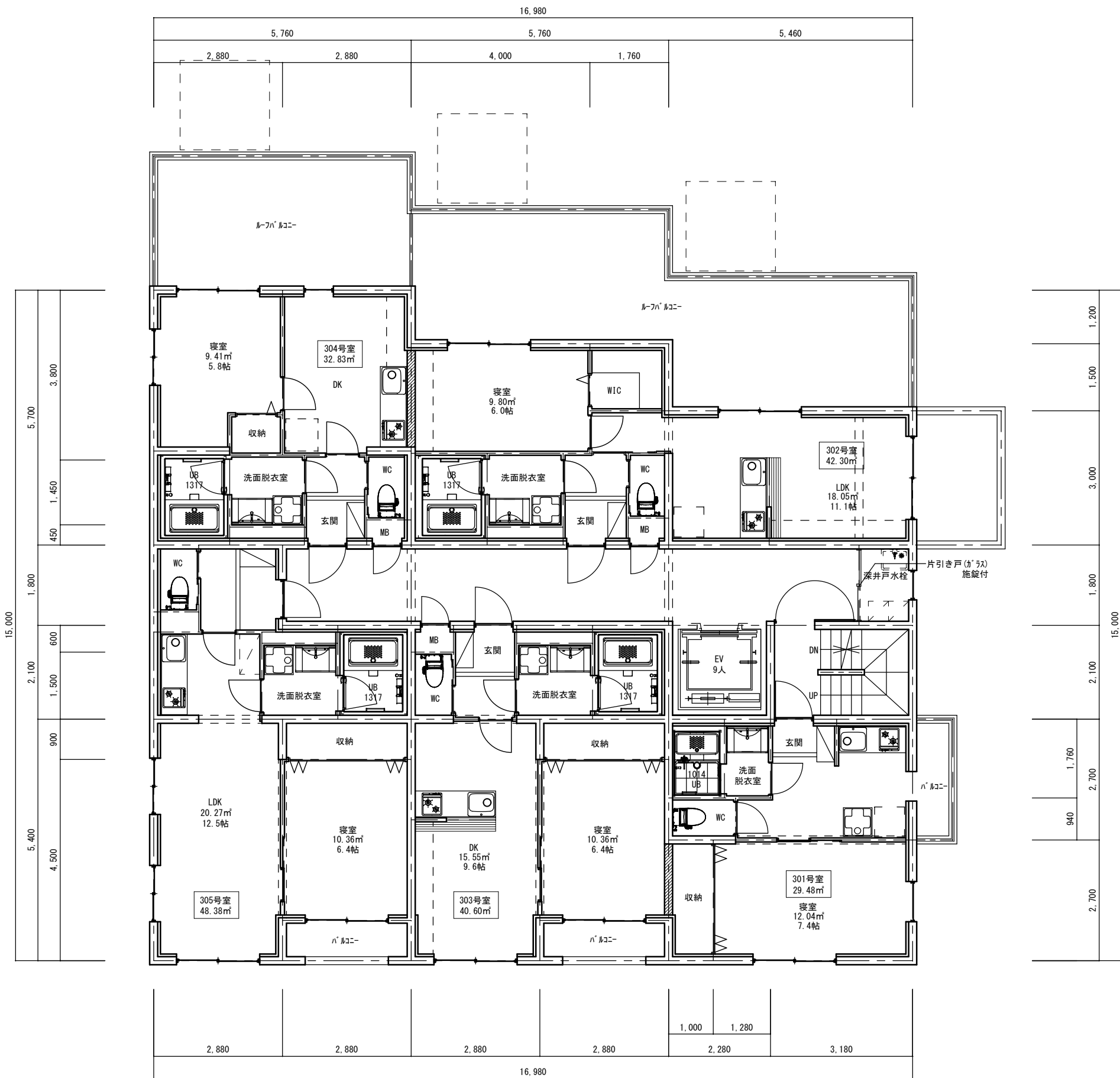
3 階 平 面 図
