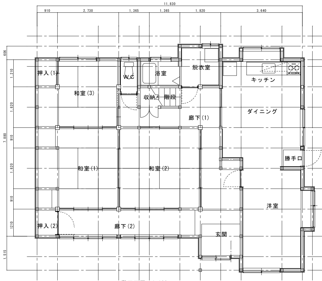
1階平面図 1:100
