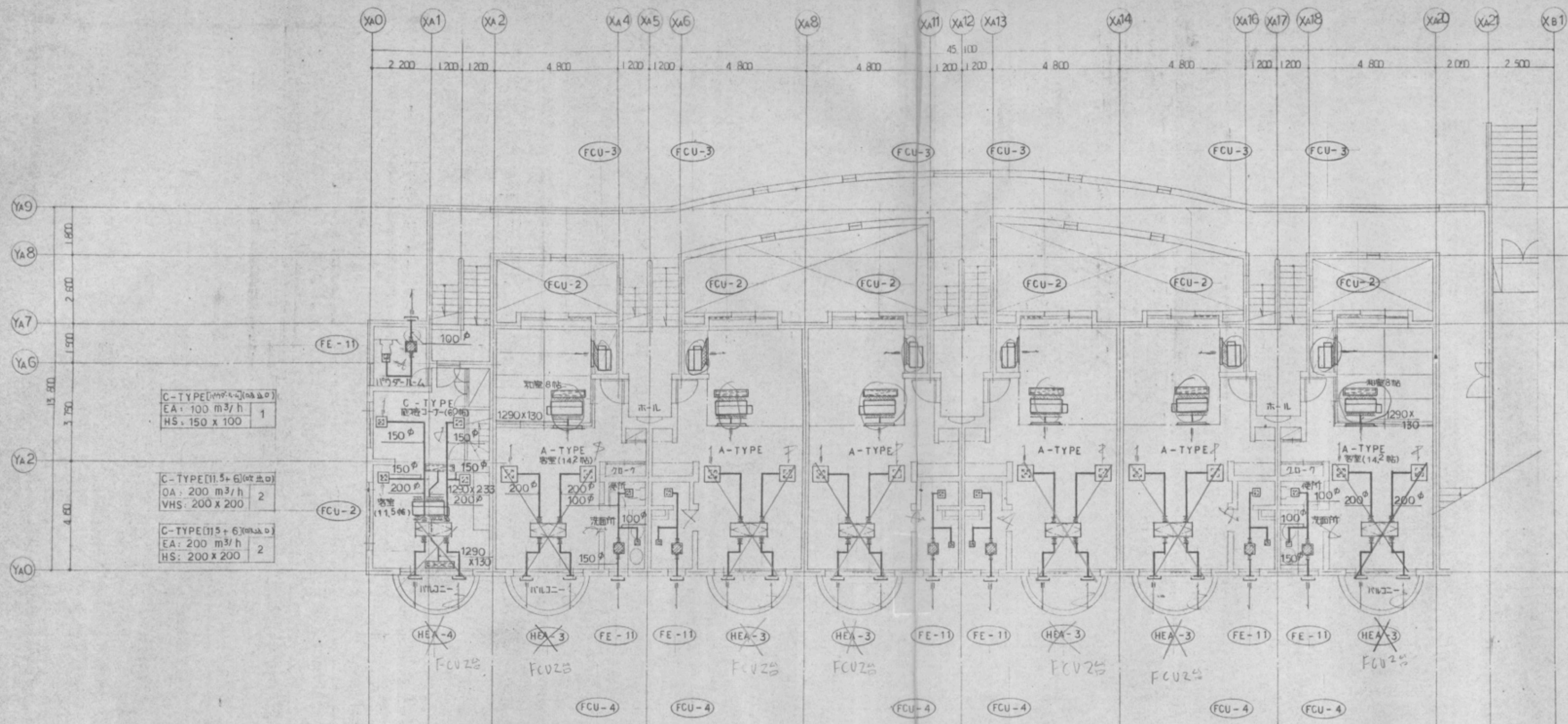
2階平面図 S=1:100
