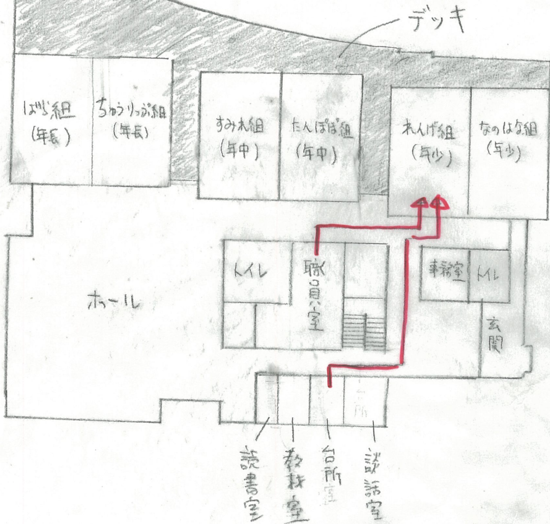
☒ 幼稚園舎の1階平面図
