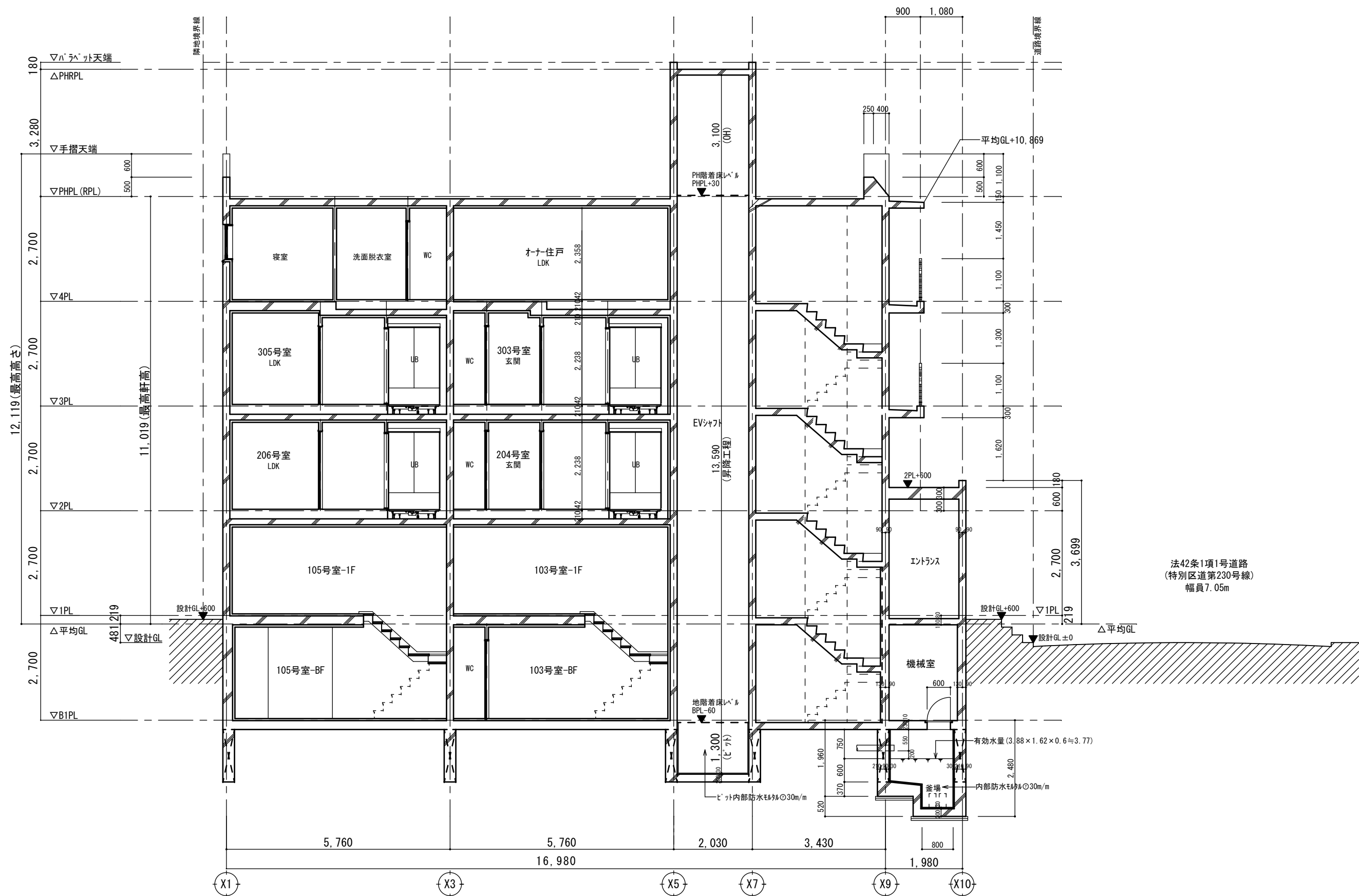
X-X' 断面図 S-1/100
