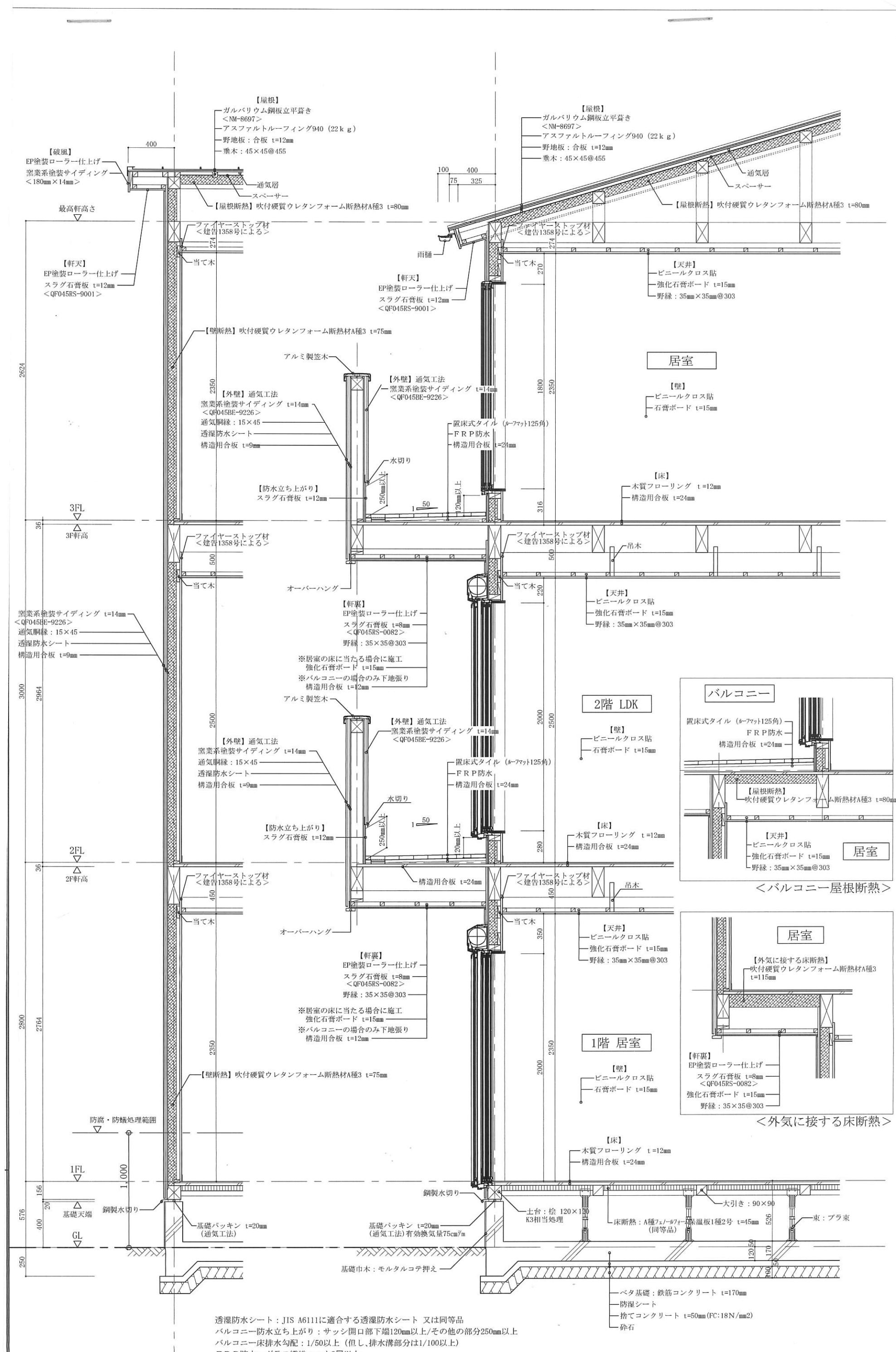
矩 計 図
