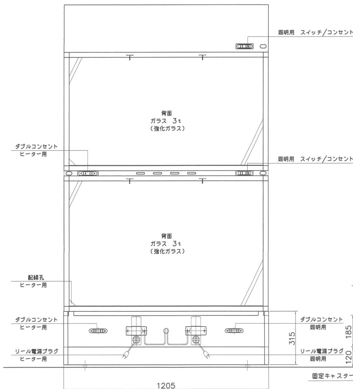
背面図
