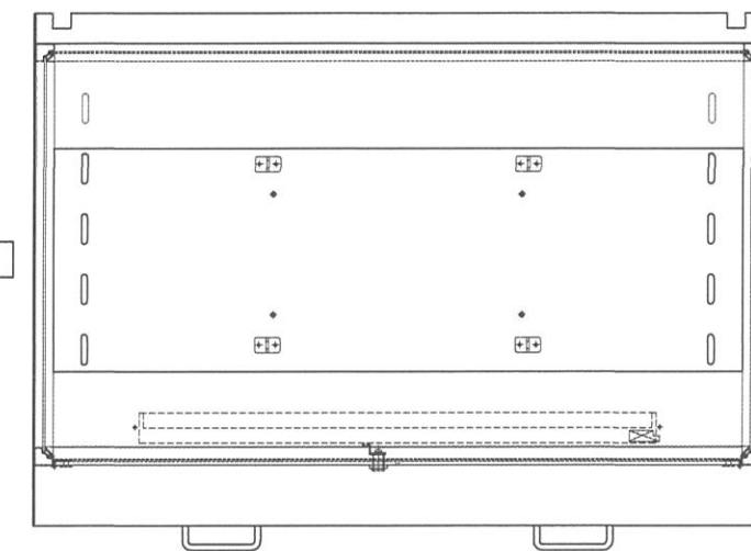
上面図
