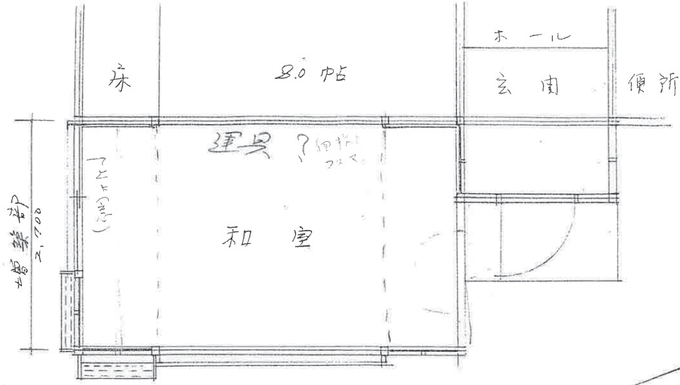
増築平面図 4.25坪
