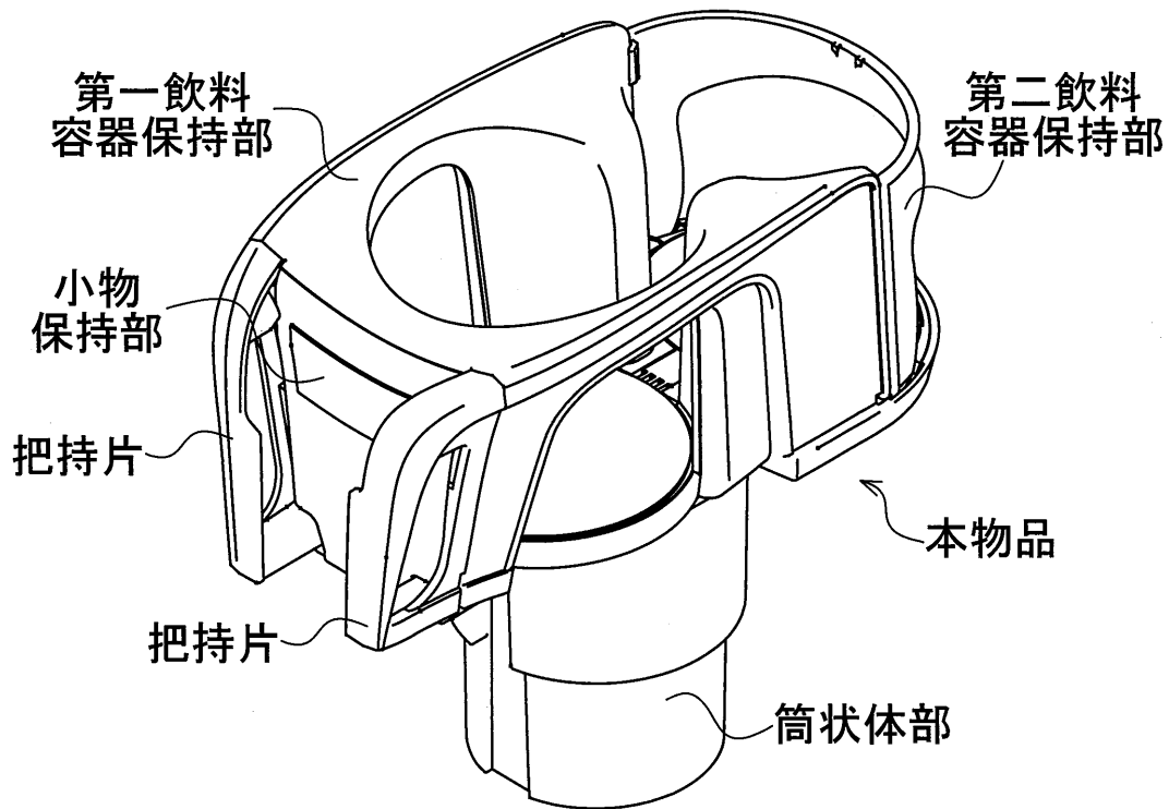
【参考斜視図】
