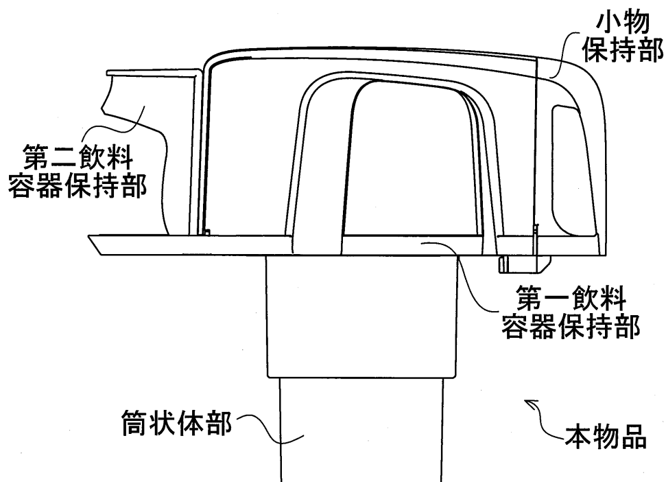
【第二变形状態を示す参考底面図】
