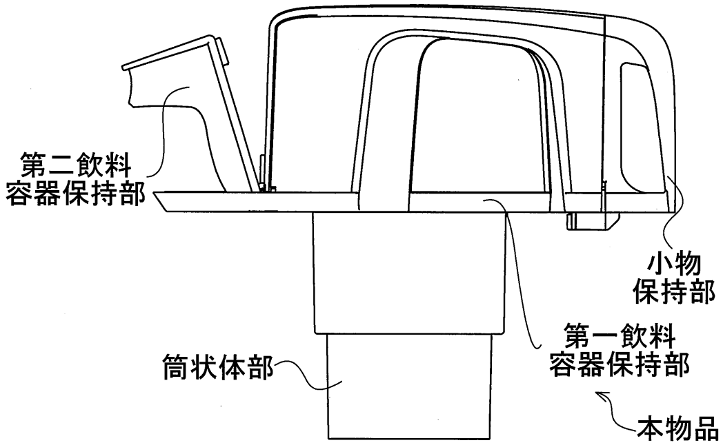
【第二飲料容器保持部の傾斜状態を示す参考左側面図】
