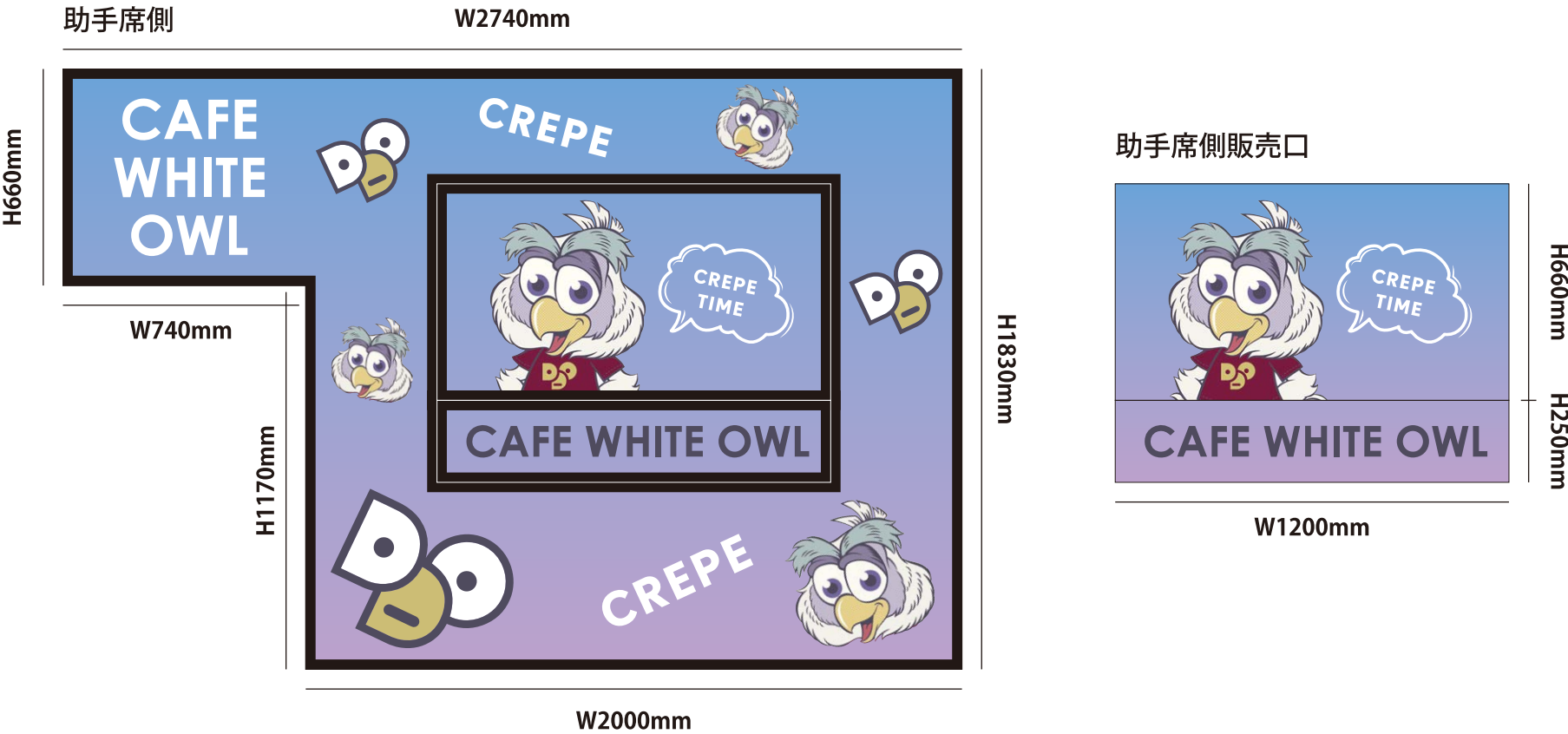
助手席側サイドカバー A案
