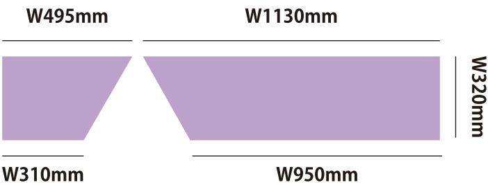
運転席側サイドカバー A案
