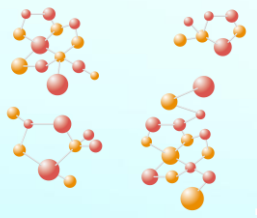
分子
