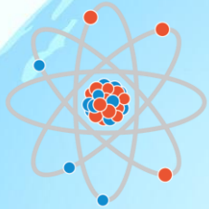
原子
