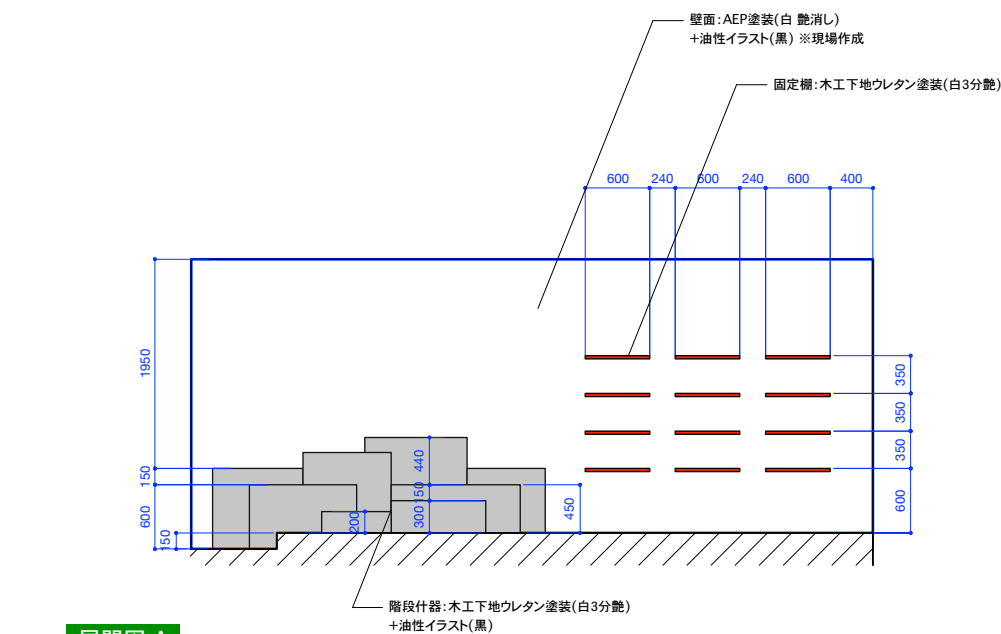
展開図 A
