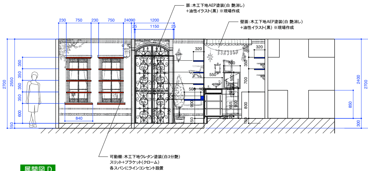
展開図 D
