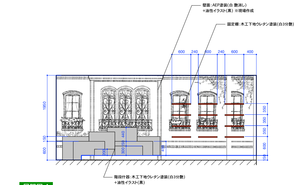
展開図 A
