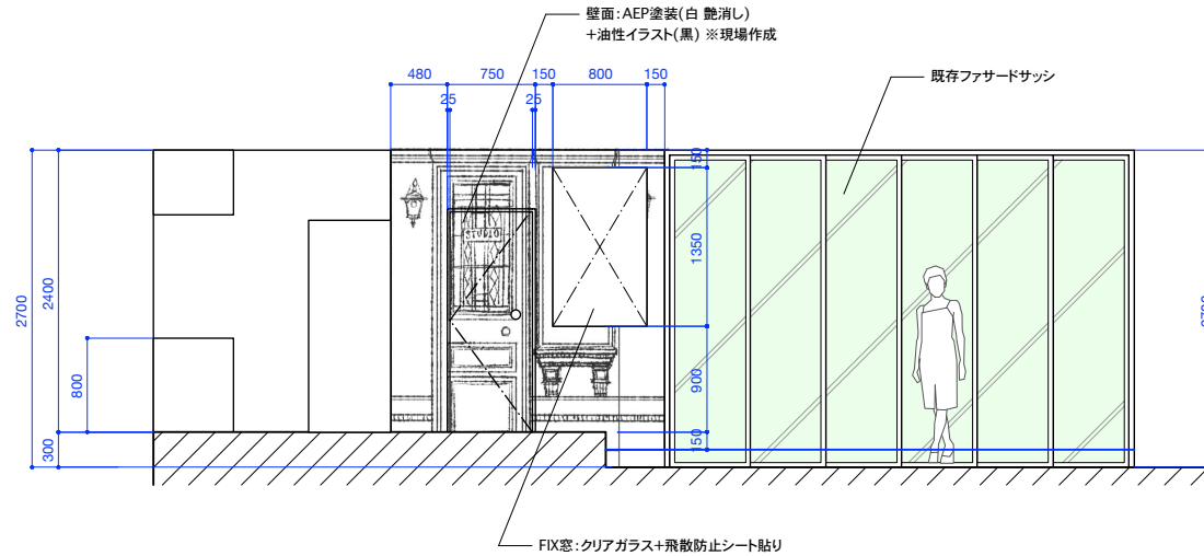
展開図 E
