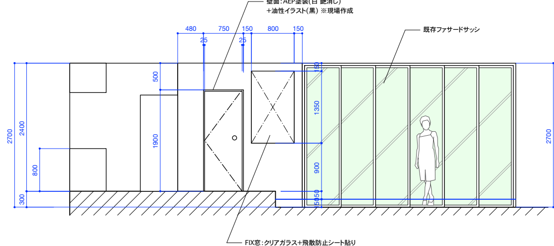
展開図 E
