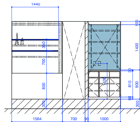
展開図 C
