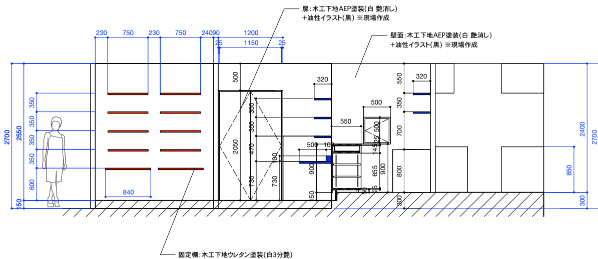
展開図 D
