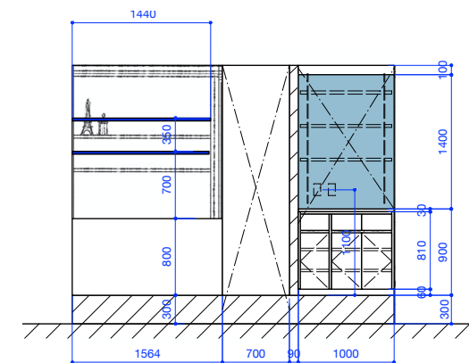
展開図 C
