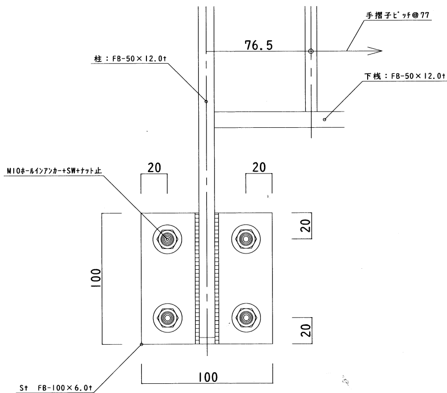
躯体取合正面図 S:1/2
