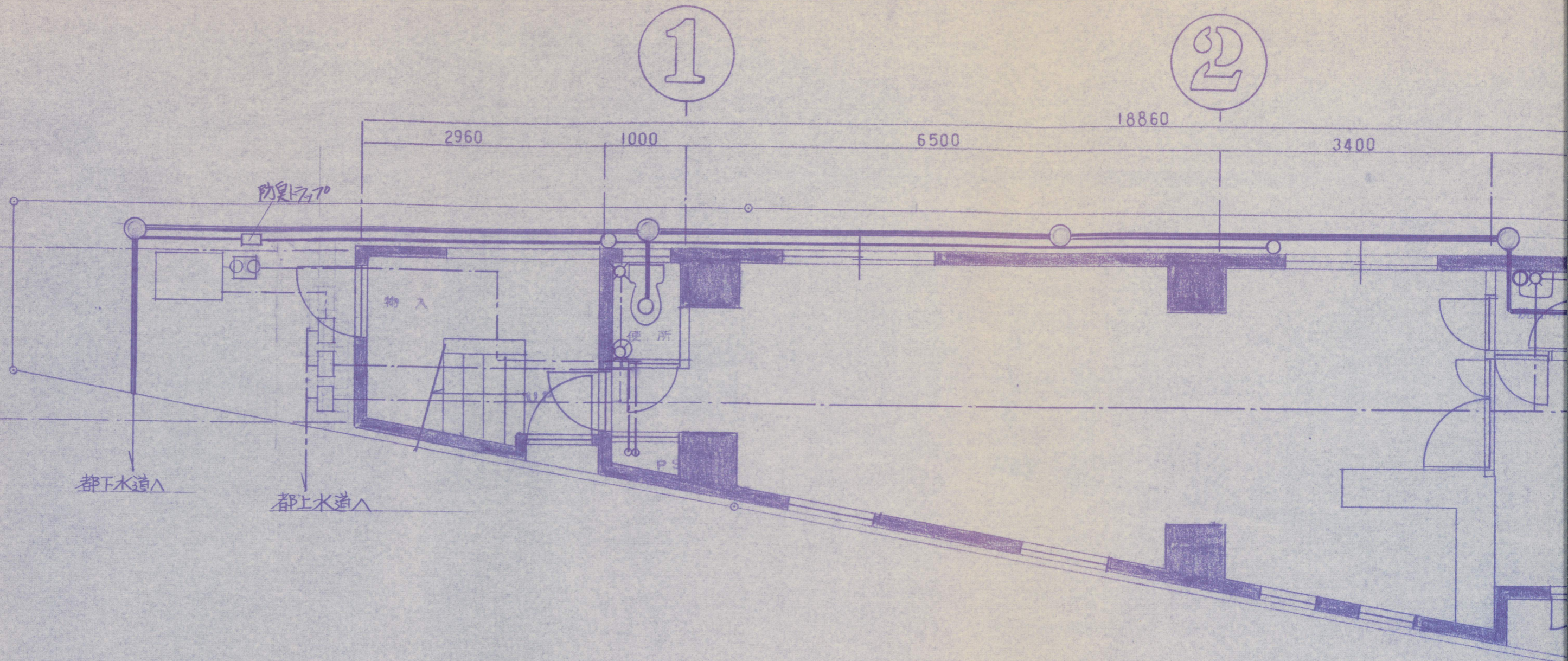
1階平面図 1/50
