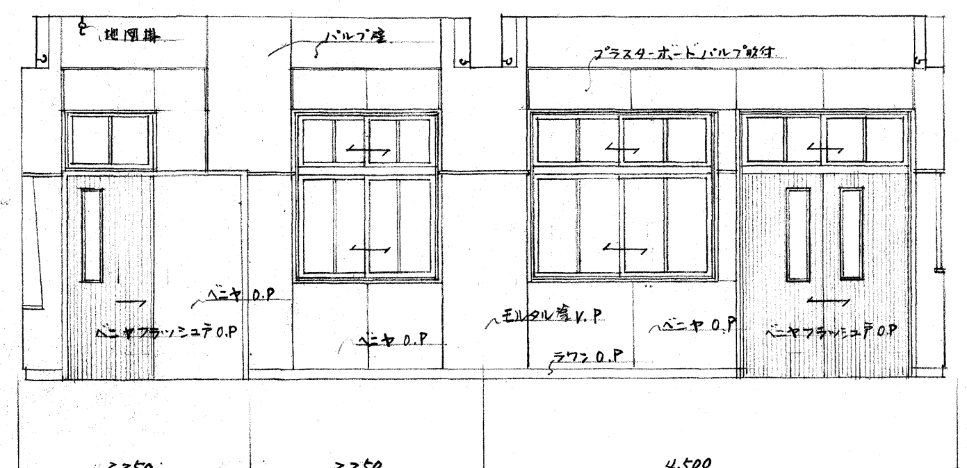
教室北側展開図 S: 1/50
