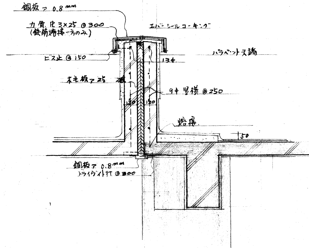
屋上天井エキスパンション詳細 S: 1/20
