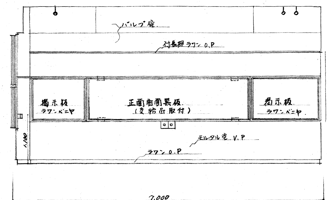
教室東側展開図 S: 1/50
