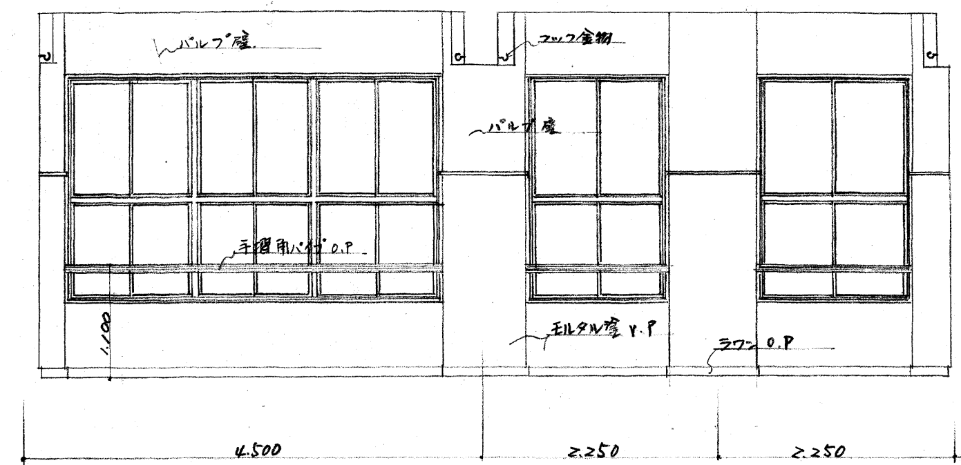
教室南側展開図 S: 1/50
