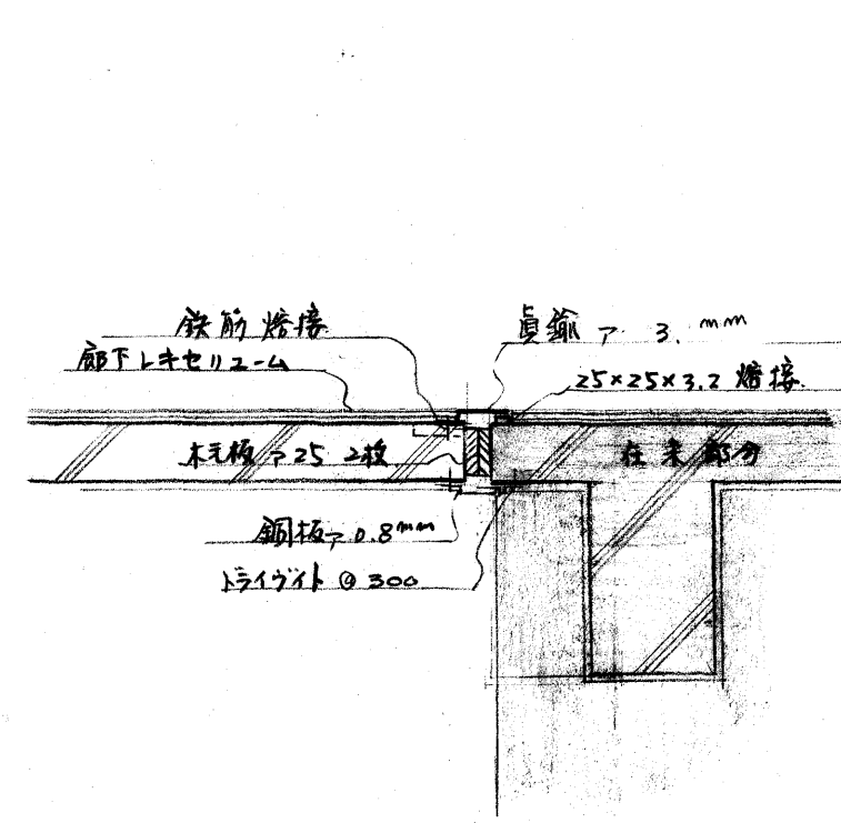
廊下床エキスパンション詳細 S: 1/20
