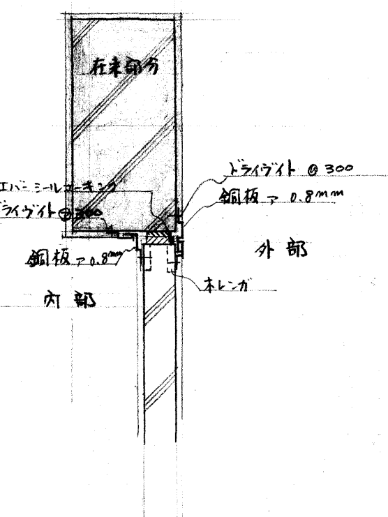
内外壁エキスパンション断面詳細 S: 1/20
