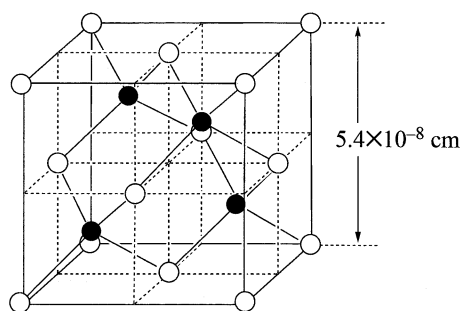
図 1. ケイ素の結晶構造
