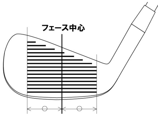
(図2)フェース中心の決定(アイアン系)
