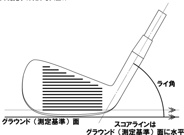
(図3)アイアン系ライ角基準
