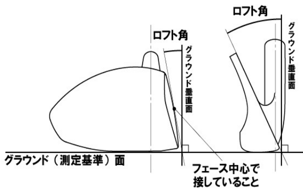
(図3)ロフト角基準
