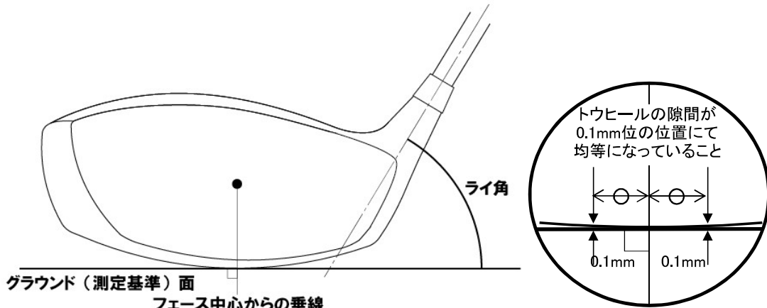
(図2)ウッド系ライ角基準
