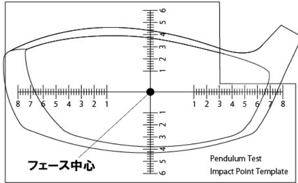
(図1)フェース中心の決定(ウッド系)
