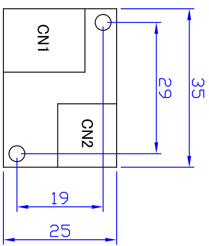
基板 FR-4 t=1.6
