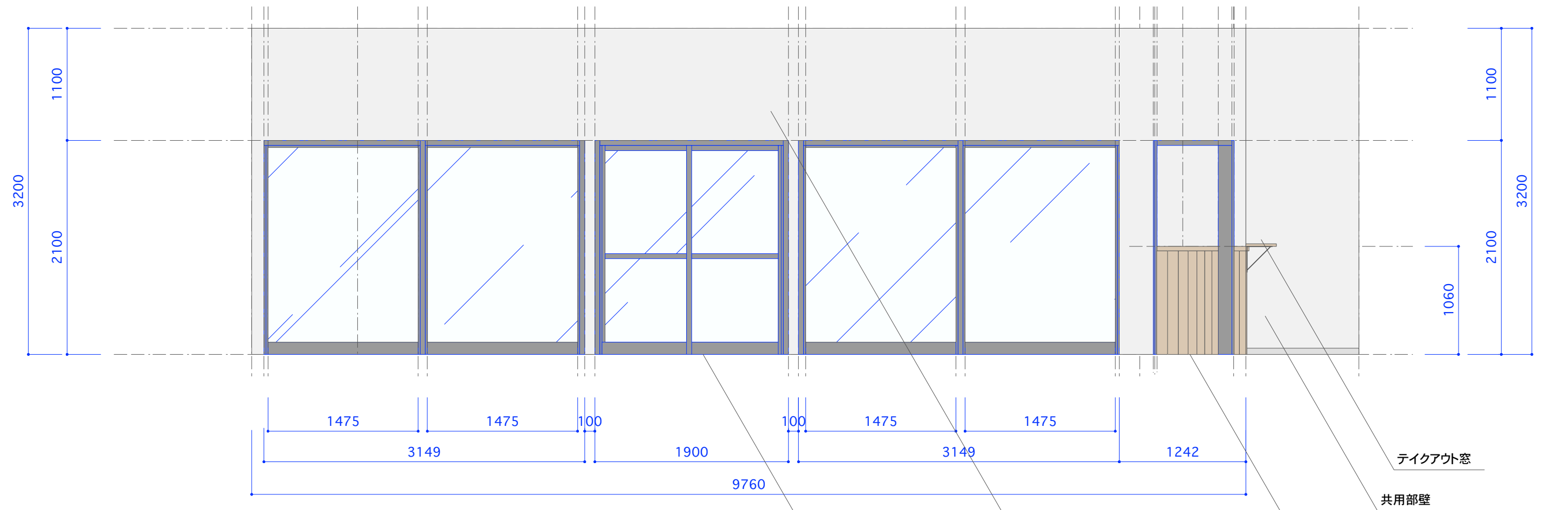
【B立面図】
