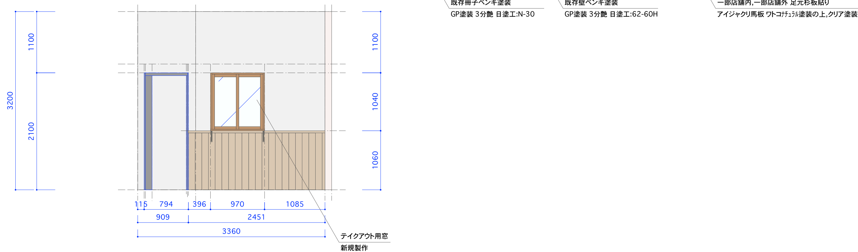
【B立面図】
